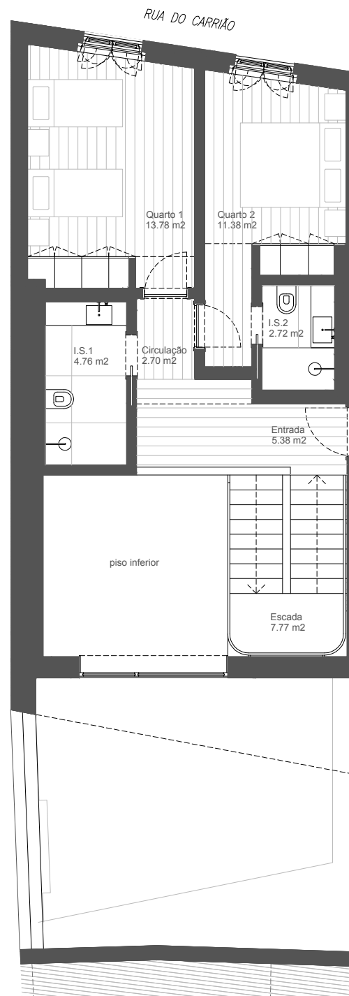
PLANTA NÍVEL 2 ESCALA 1:100
