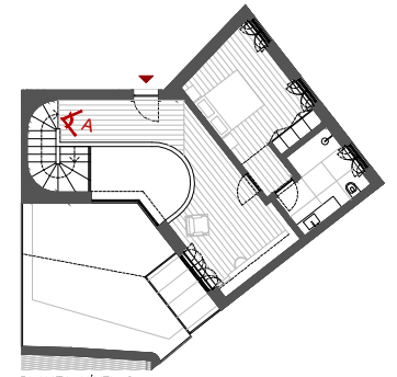
PLANTA NIVEL 2
