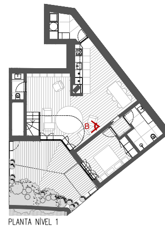
PLANTA NIVEL 1
