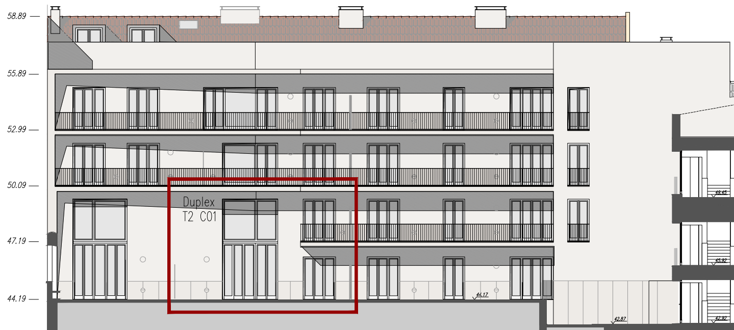
ALÇADO PÁTIO / LOGRADOURO INTERIOR ESCALA 1:200
