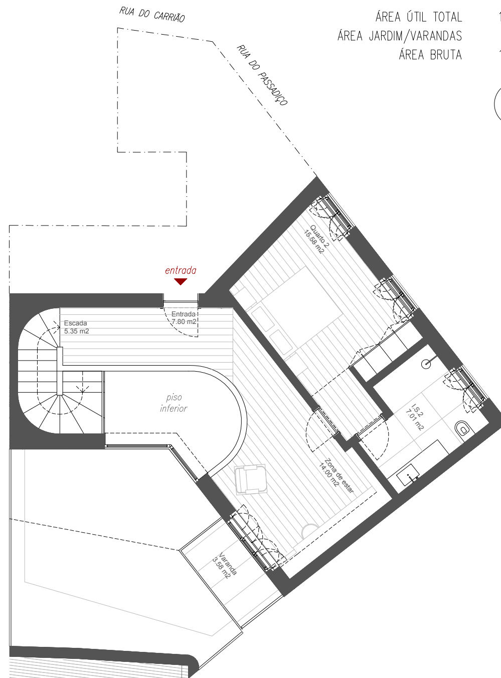
PLANTA NÍVEL 2 ESCALA 1:100
