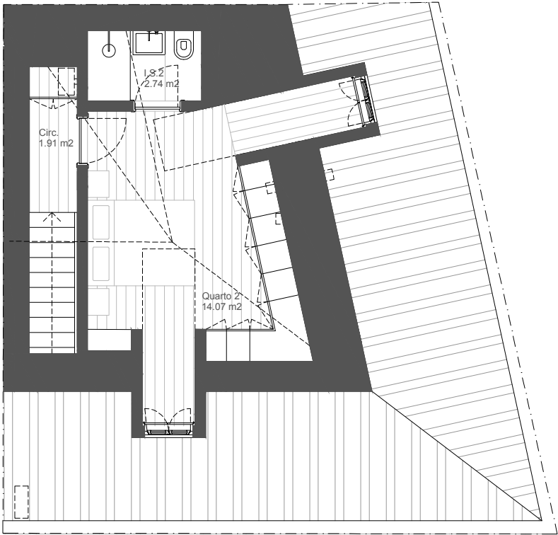
PLANTA NÍVEL 4 ESCALA 1:100
