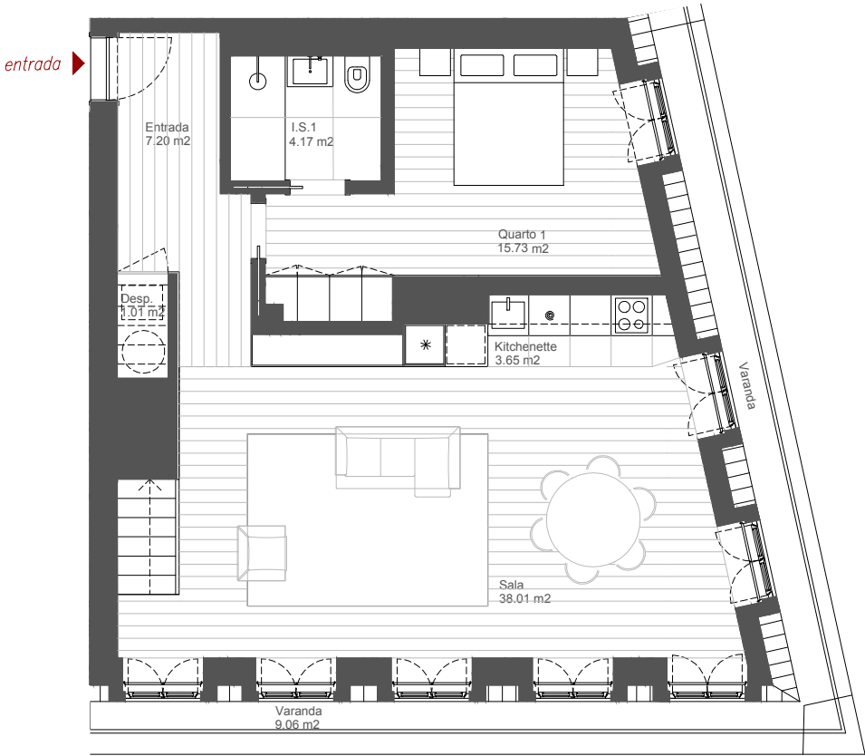
PLANTA NÍVEL 3 ESCALA 1:100
