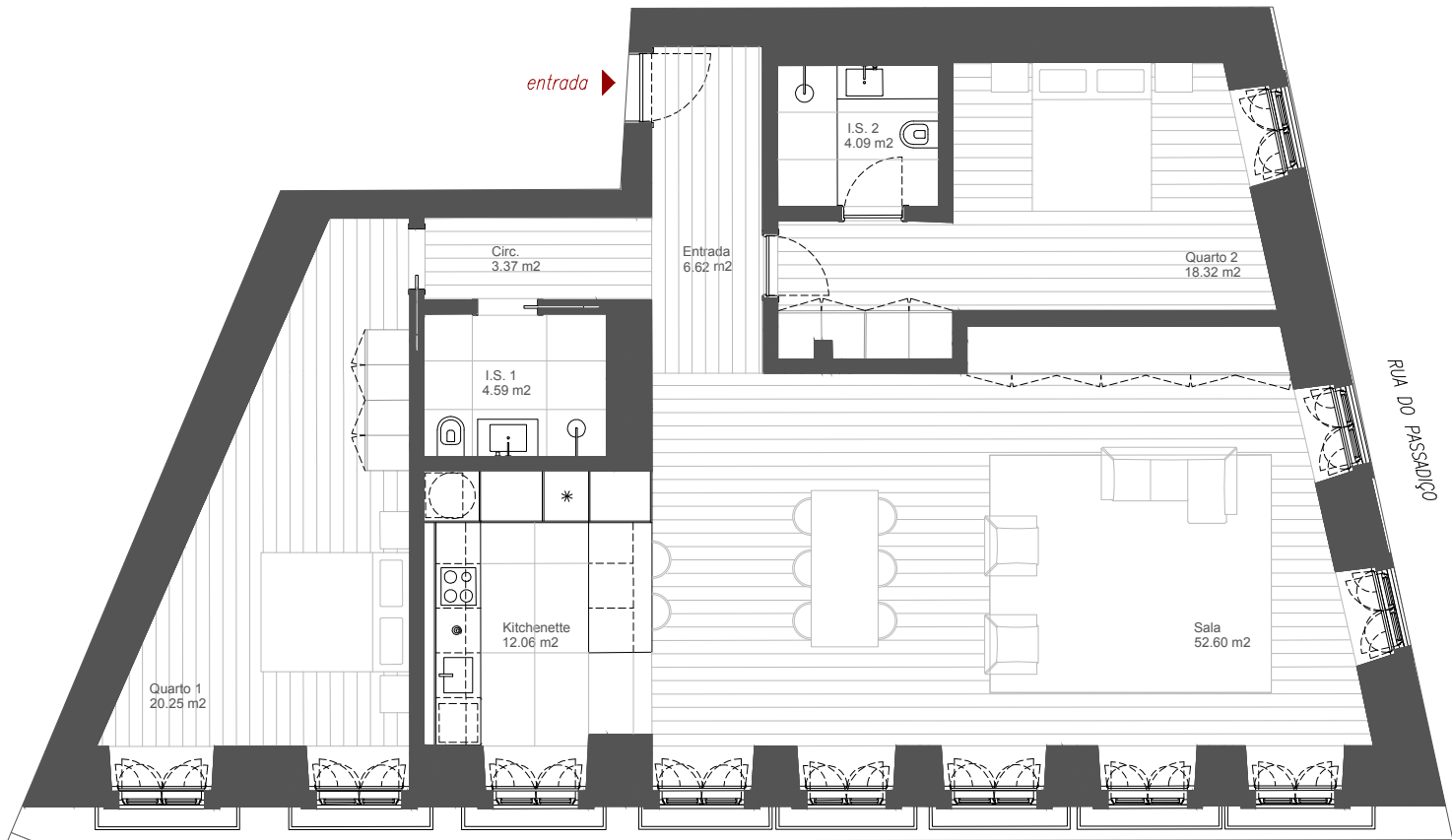
PLANTA NÍVEL 2 ESCALA 1:100
