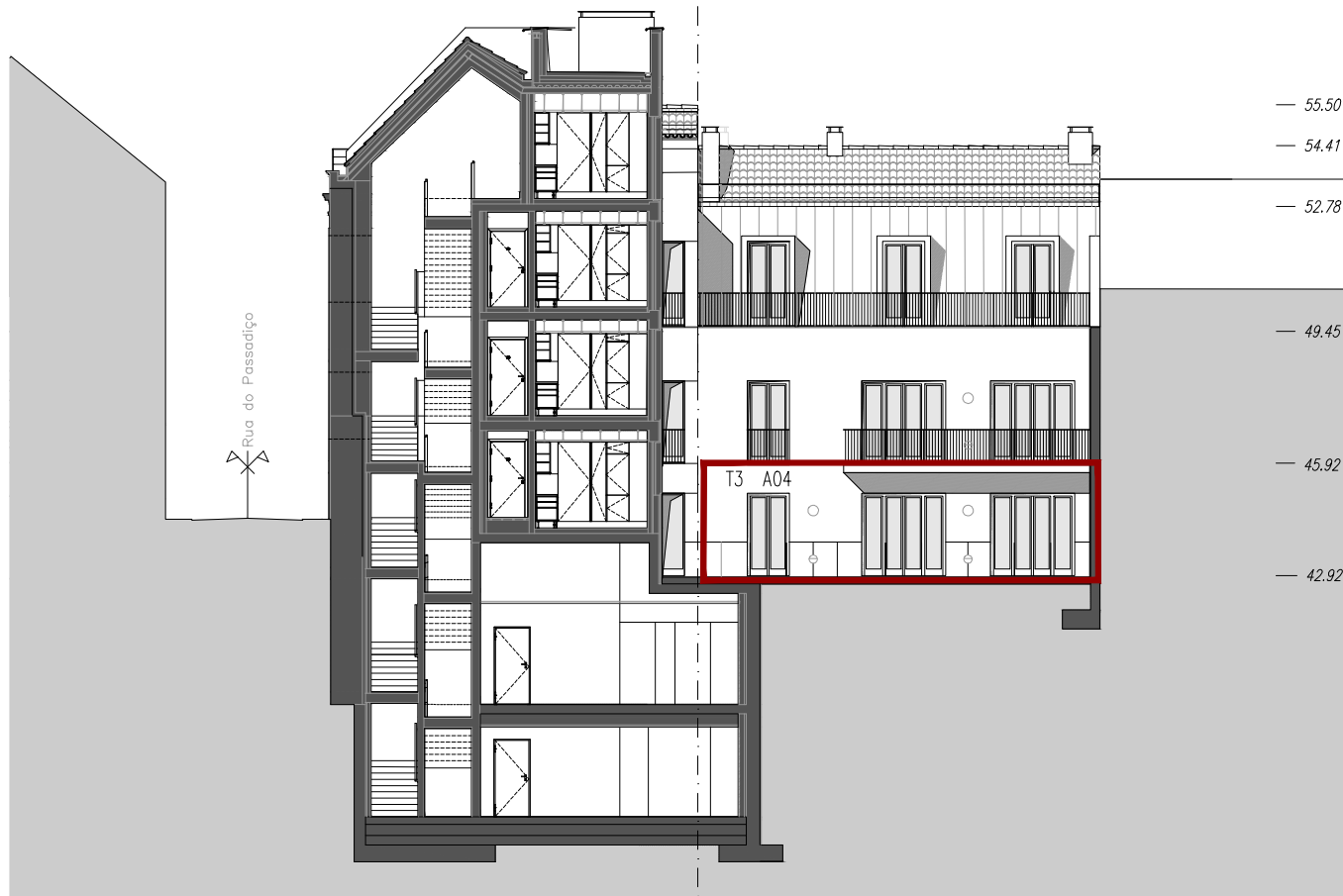
CORTE DD / ALÇADO LOGRADOURO INTERIOR ESCALA 1:200
